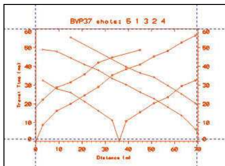
Fig.3- Dromocrona correspondiente a un perfil genérico
