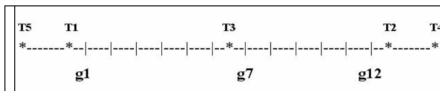
Fig. 1-Disposición de los puntos de disparo, offset y geófonos para tendidos sísmicos de 5 tiros.
