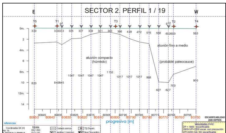
Fig.5- Perfil geosísmico correspondiente al Sector2 de la traza.
