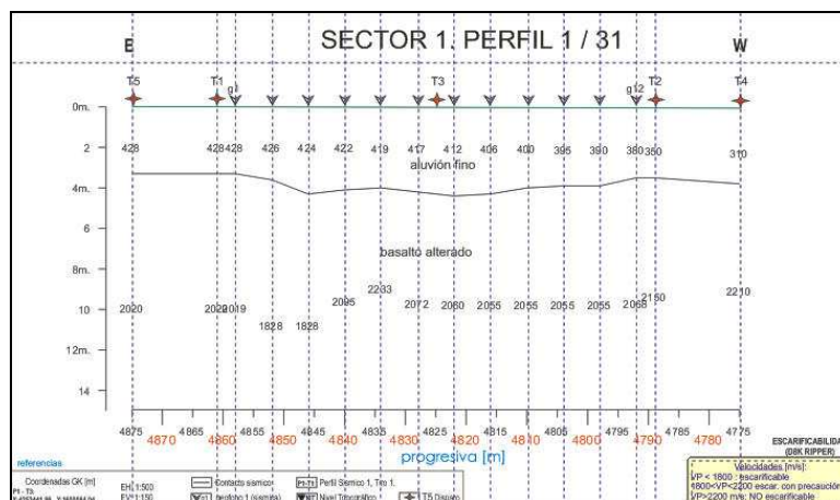
Fig.4- Perfil geosísmico típico correspondiente al Sector1 de la traza.
